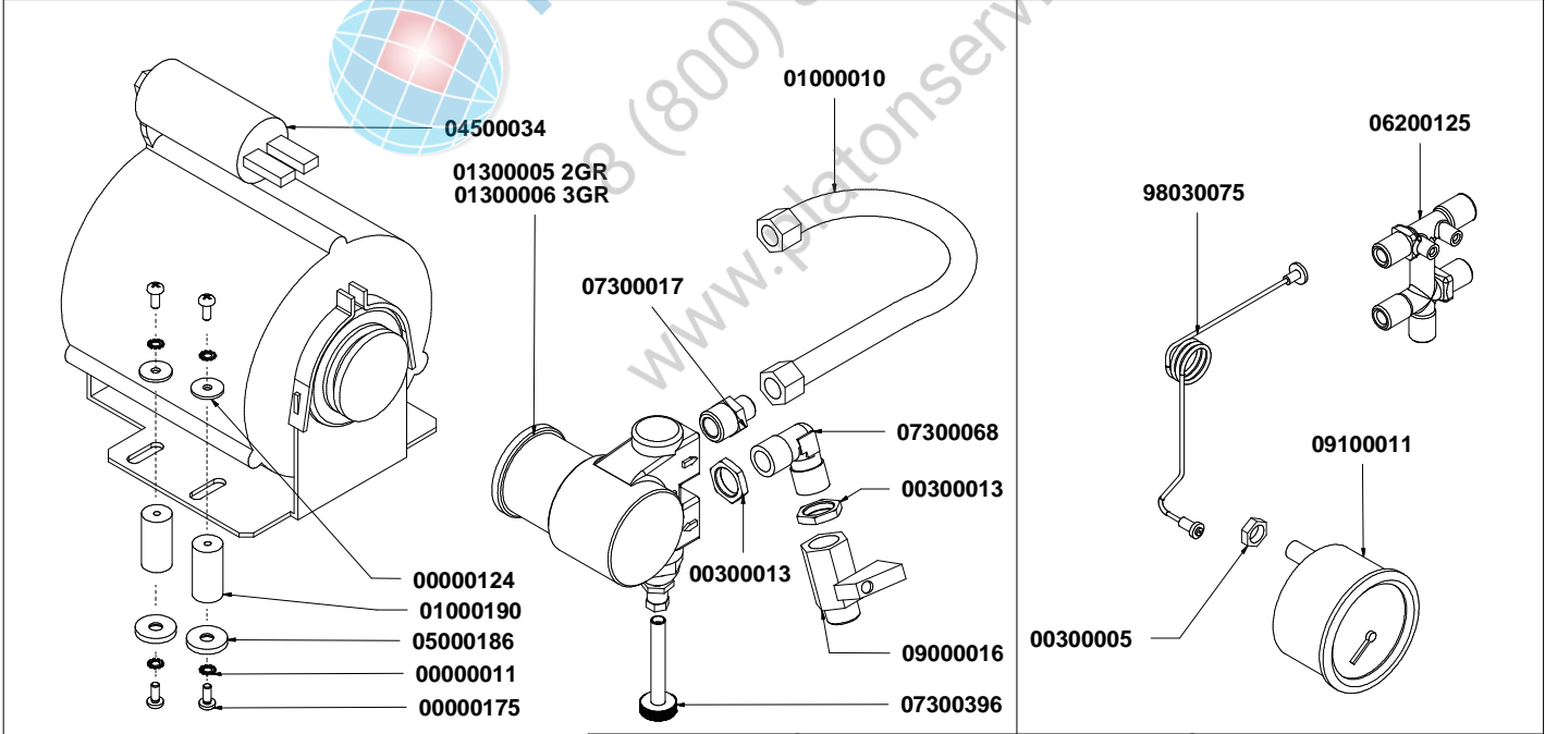
Componenti idraulici Hydraulic Components
